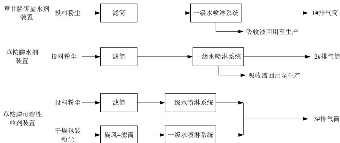
图 4.2.1-1 项目废气污染物治理措施示意图
