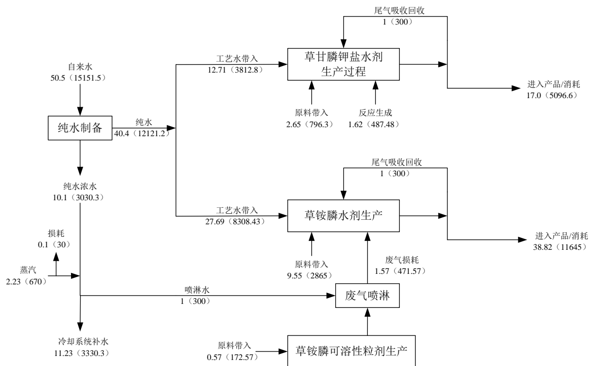
图 3.6-1 项目实际水平衡图 单位: t/a
