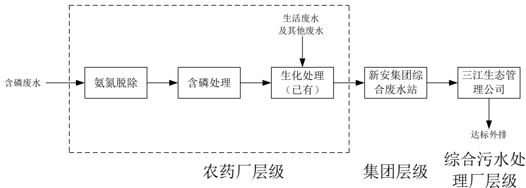
图 4.1.2-1 农药厂污水处理层级示意图
