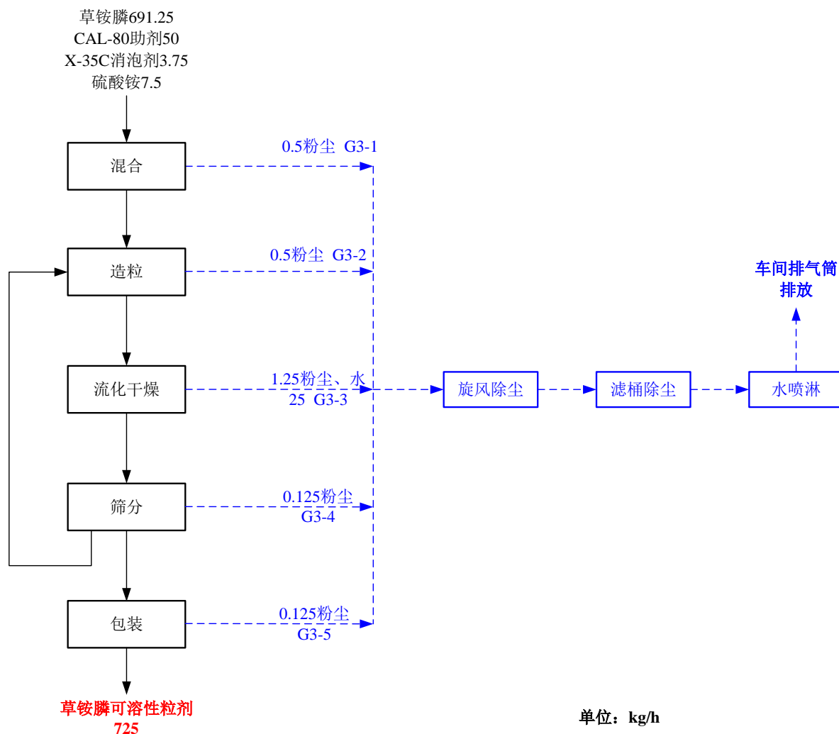
图 3.5.2-1 草铵膦可溶性粒剂原药生产工艺流程和产污位置图
