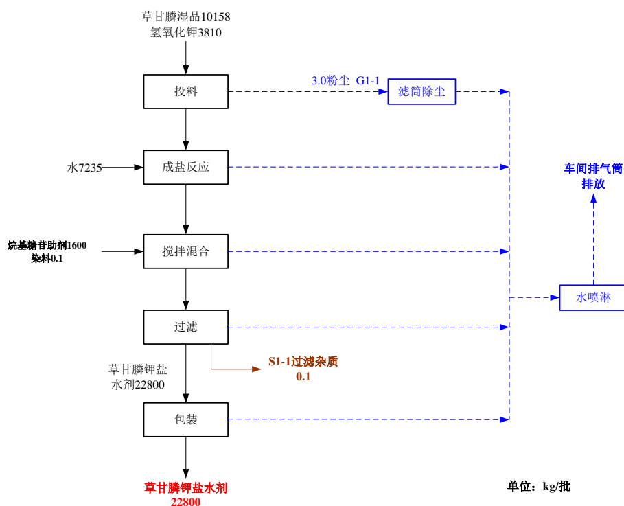
图 3.5.1-1 草甘膦钾盐生产工艺流程及产污位置图
