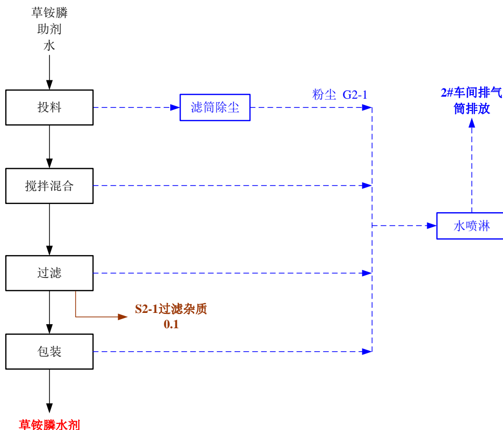
图 3.5.1-2 草铵膦水剂生产工艺流程和产污位置图
